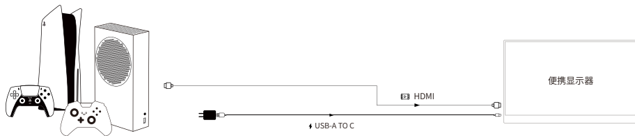
☆HDMI端口连接PS4/PS5/XBOX接线示意图
