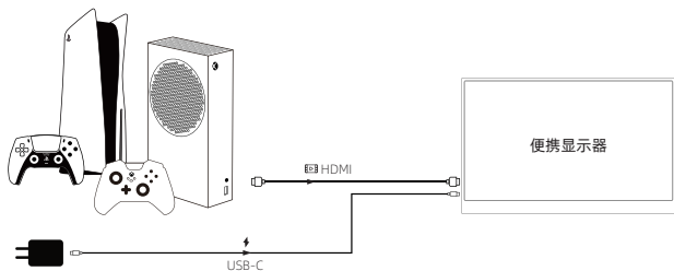
☆HDMI端口连接PS4/PS5/XBOX接线示意图
